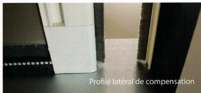
MP40 Moustiquaire coulissante latérale
